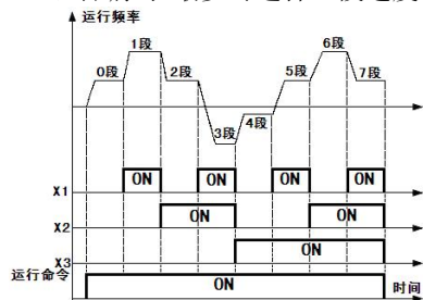
图 6-20 多段频率运行逻辑图
