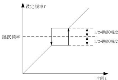
图 6-14 跳跃频率示意图
