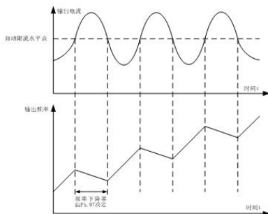
图 6-23 过流失速功能
