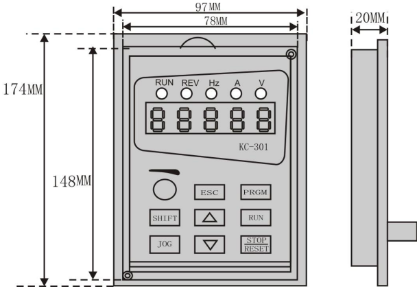
KC301 键盘开孔尺寸：148MM*78MM
