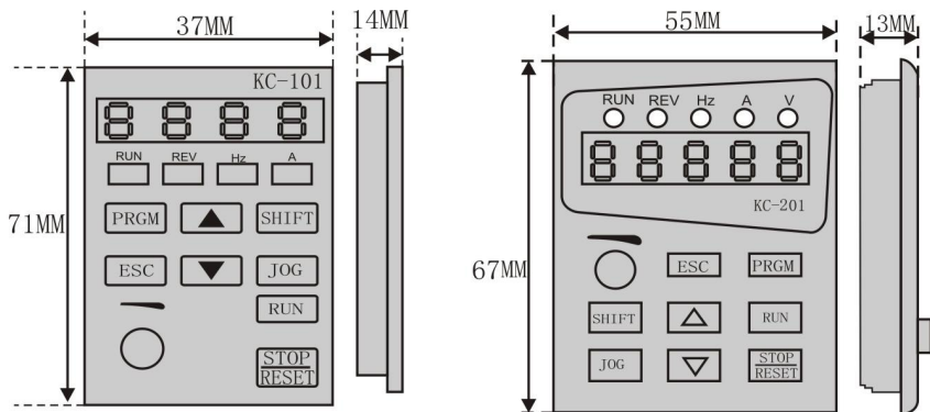
KC101 键盘开孔尺寸：37MM*71MM；
