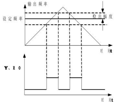
图 6-17 频率到达检出幅值示意图
