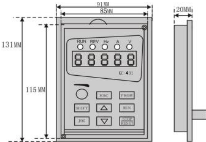
KC401 键盘开孔尺寸：116MM*86MM
